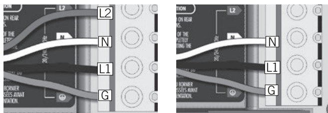
240 V (4 wires)
