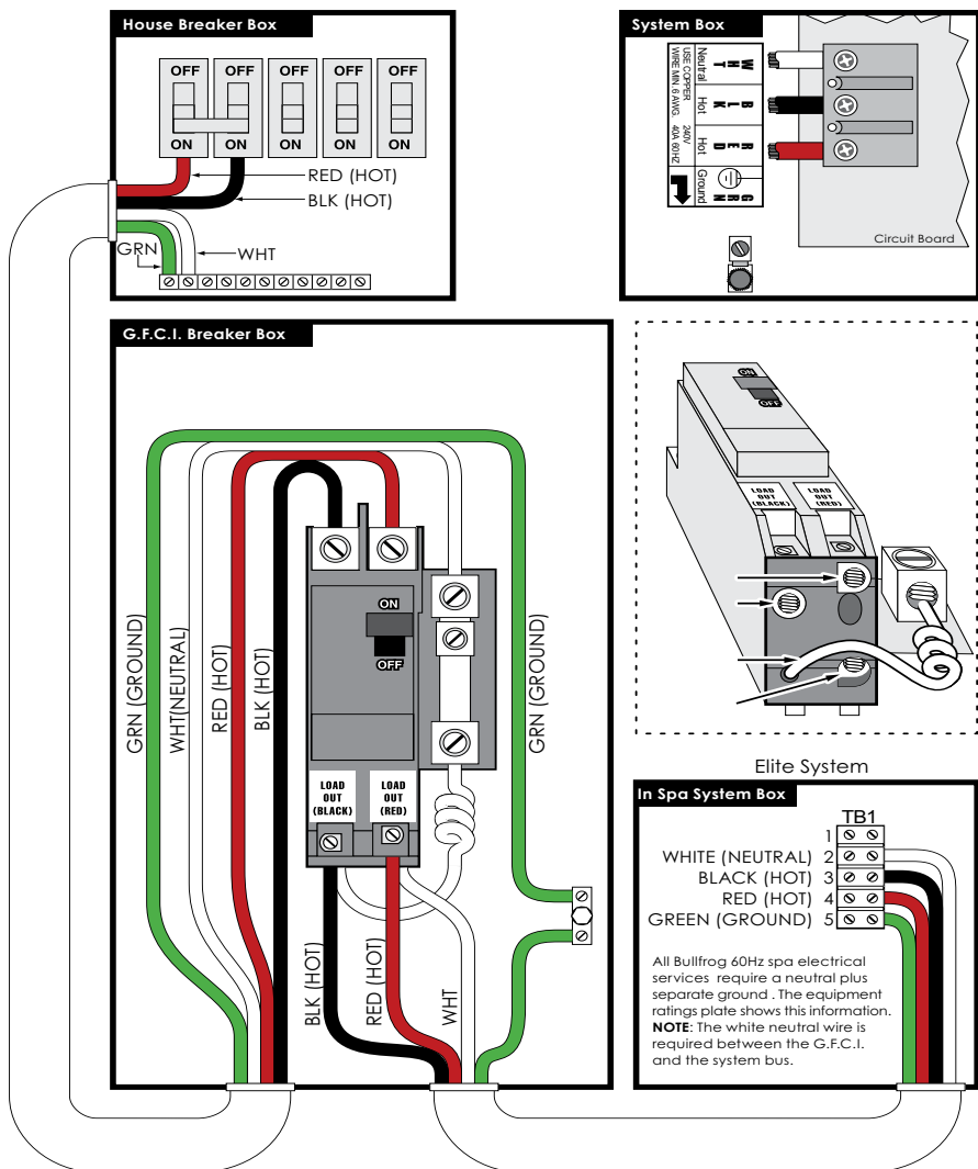
Installation typique 60Hz U.S. et Canada pour BF02, BF03 et BF05
