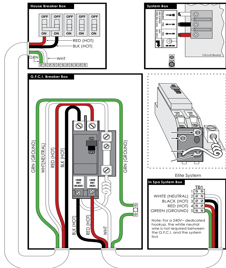
Installation typique 60Hz U.S. et Canada pour BF01, BF02 et BF03
